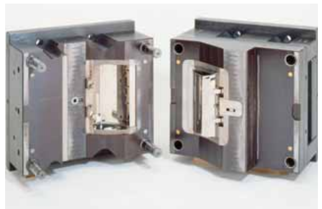
1-fach Spritzwerkzeug hochglanzpoliert
